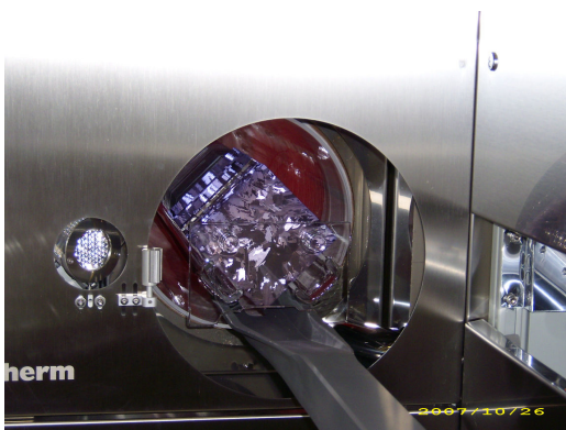
POCl 3 -Diffusion
